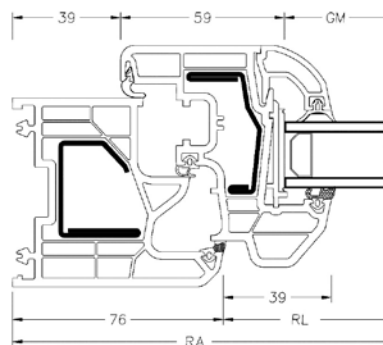
Schnitt waagrecht
