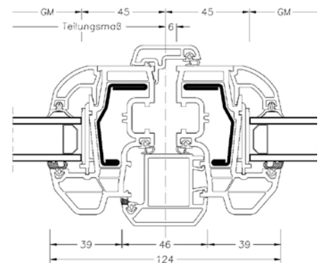
Schnitt Stulp
