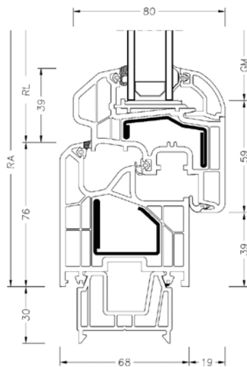
Schnitt senkrecht
